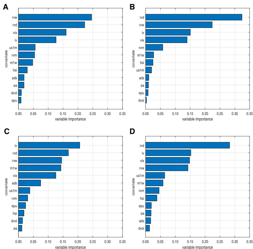
Figure 7 VI measure. (A) HAR-X. (B) EN. (C) RF. (D) NN_2^{10} .
